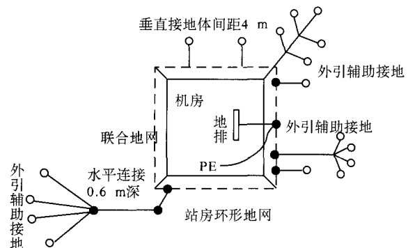
图5 站房共用接地网布设示意图
